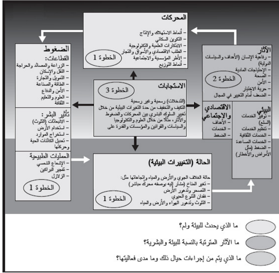
شكل (3): الإطار التحليلي المبسط لتقييم البيئة المتكامل ورفع التقارير ذات الصلة
